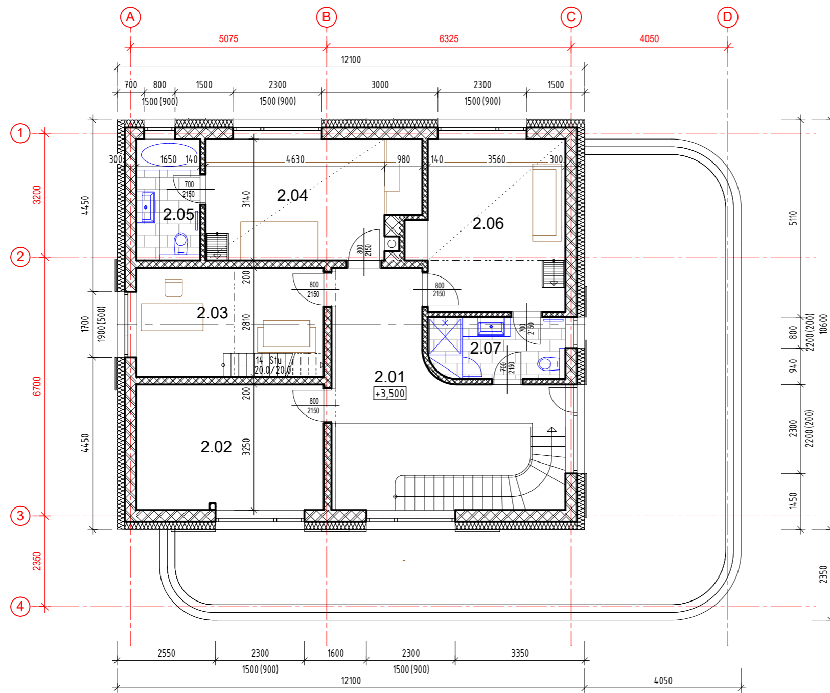
PÔDORYS 2.NP
