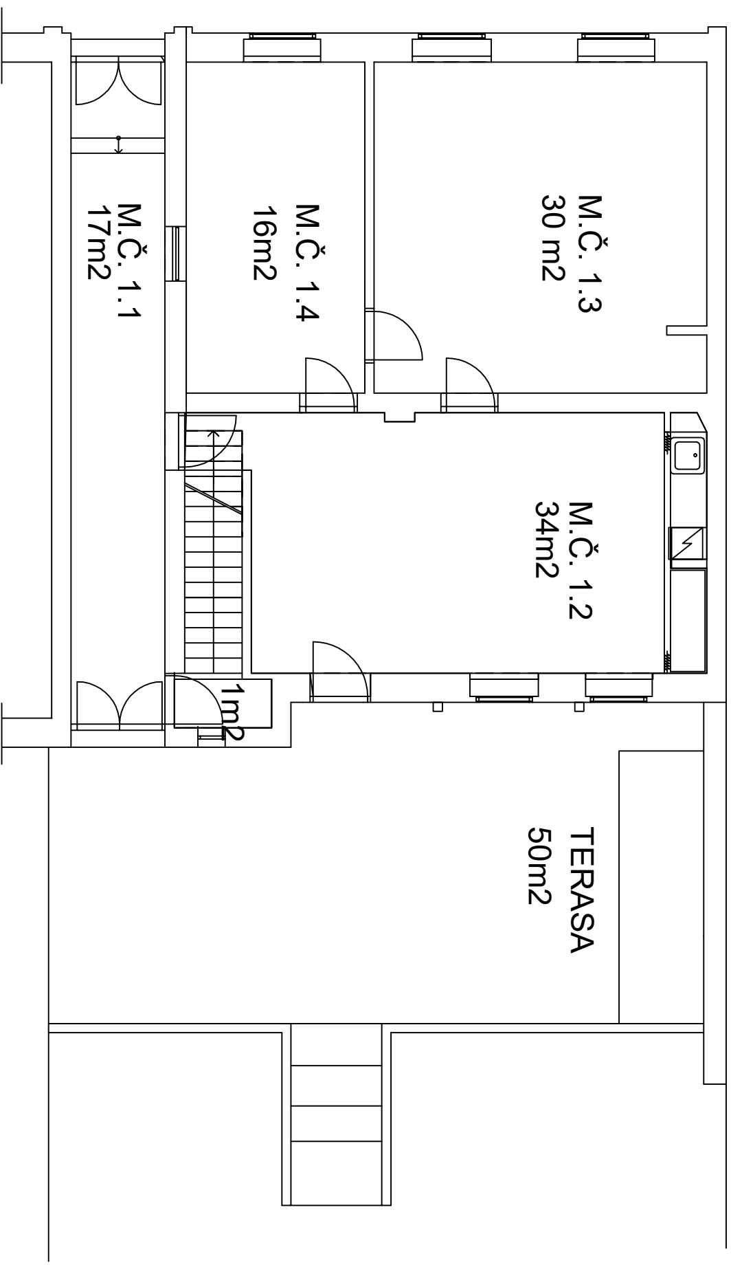
PODORYS PRÍZEMIA 97m 2
